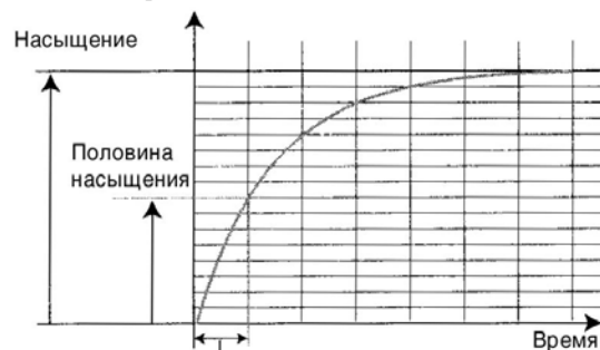
Рис. 1 График поглощения азота Уровень азота
